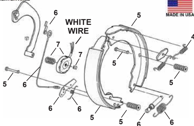
COMPLETE ASSEMBLIES F2344 (1 PAIR)
