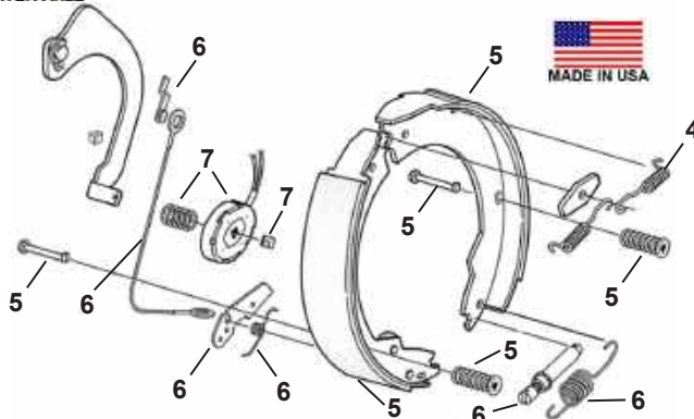
COMPLETE ASSEMBLIES F2343 (1 PAIR)
